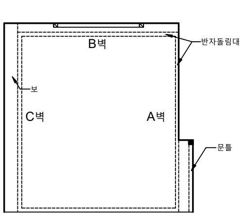
평면도
